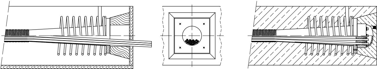
Recessed stressing anchorage SA
