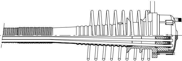
Inaccessible fixed anchorage FA 1), 2)
